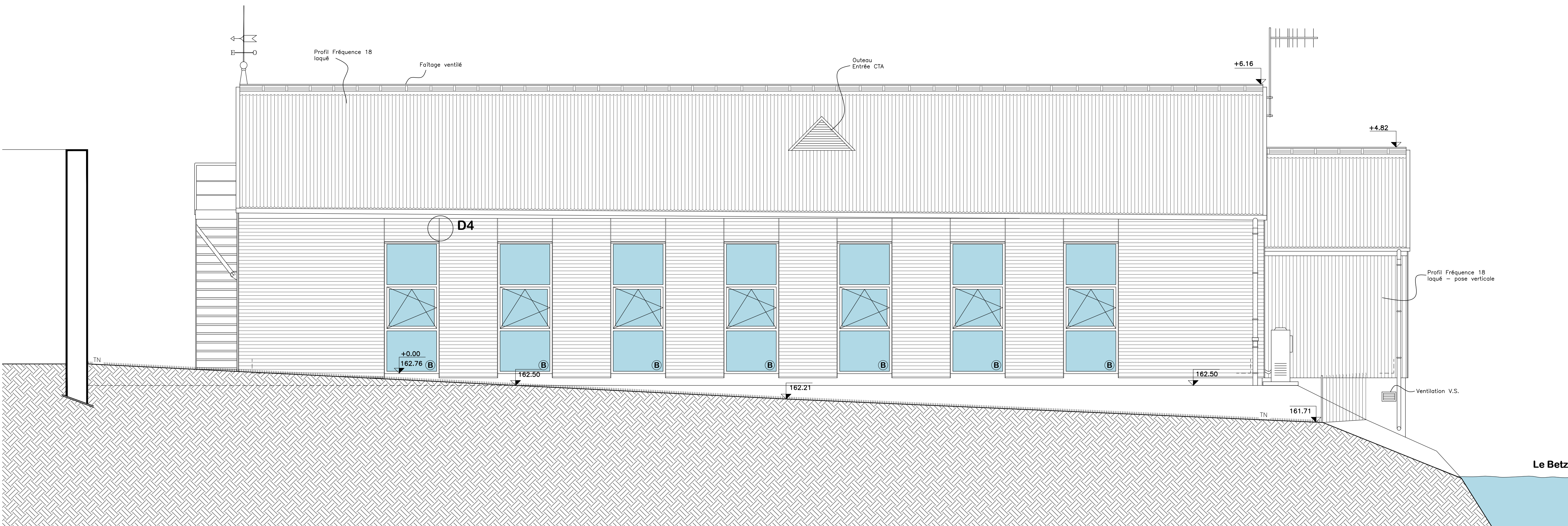
Façade Nord
