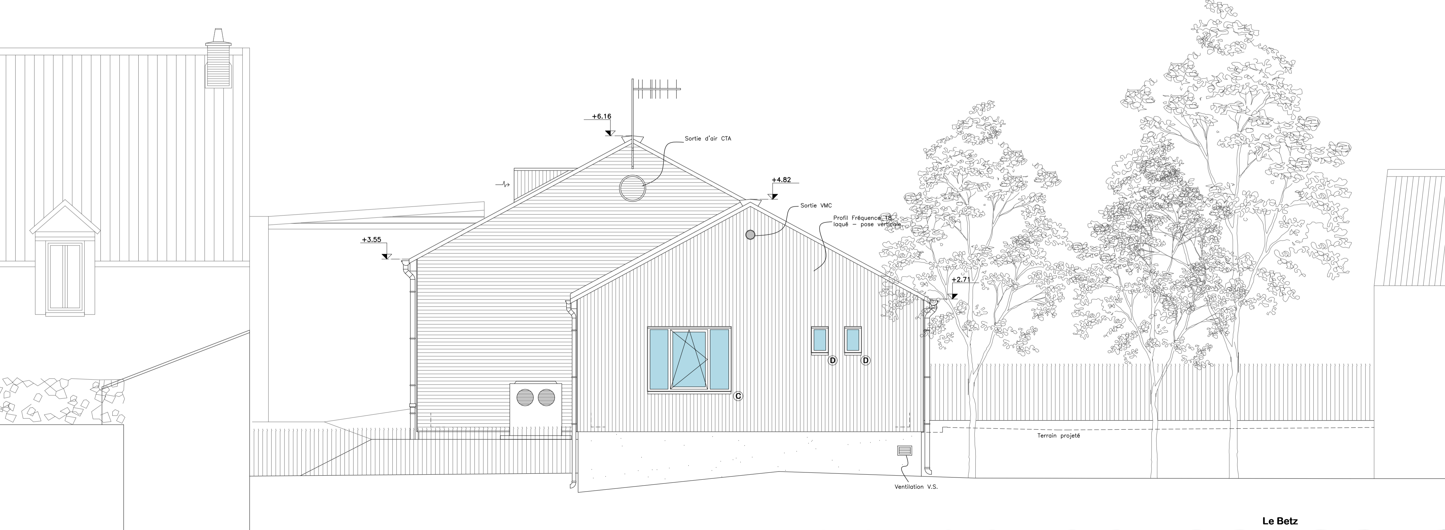
Façade Ouest
