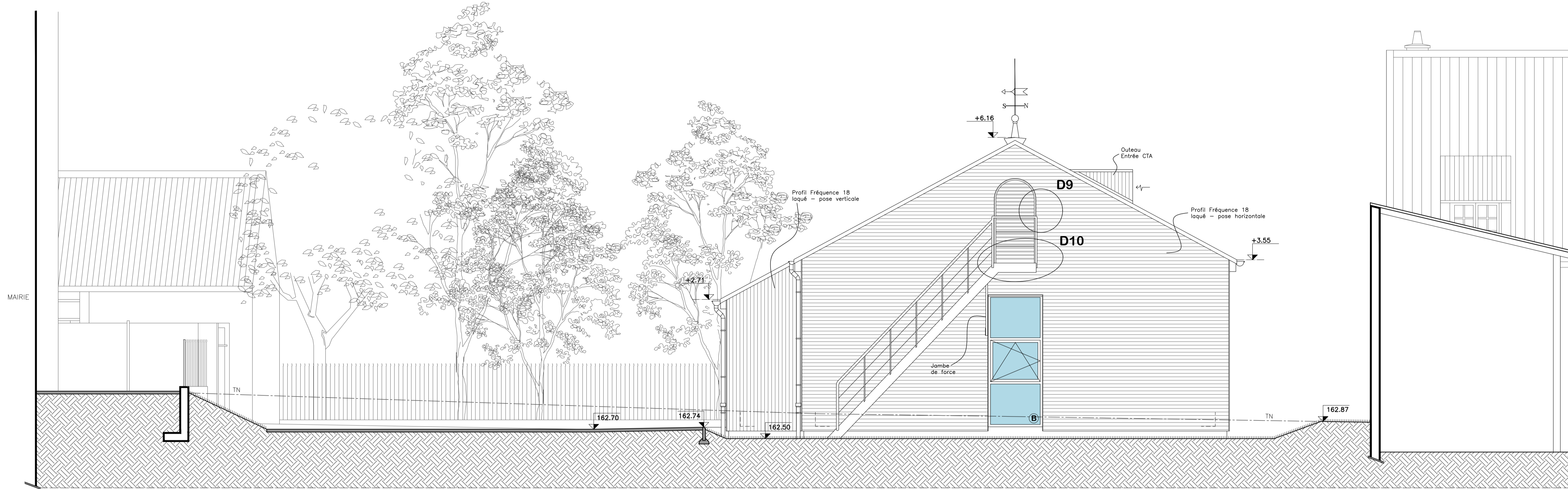
Façade Est
