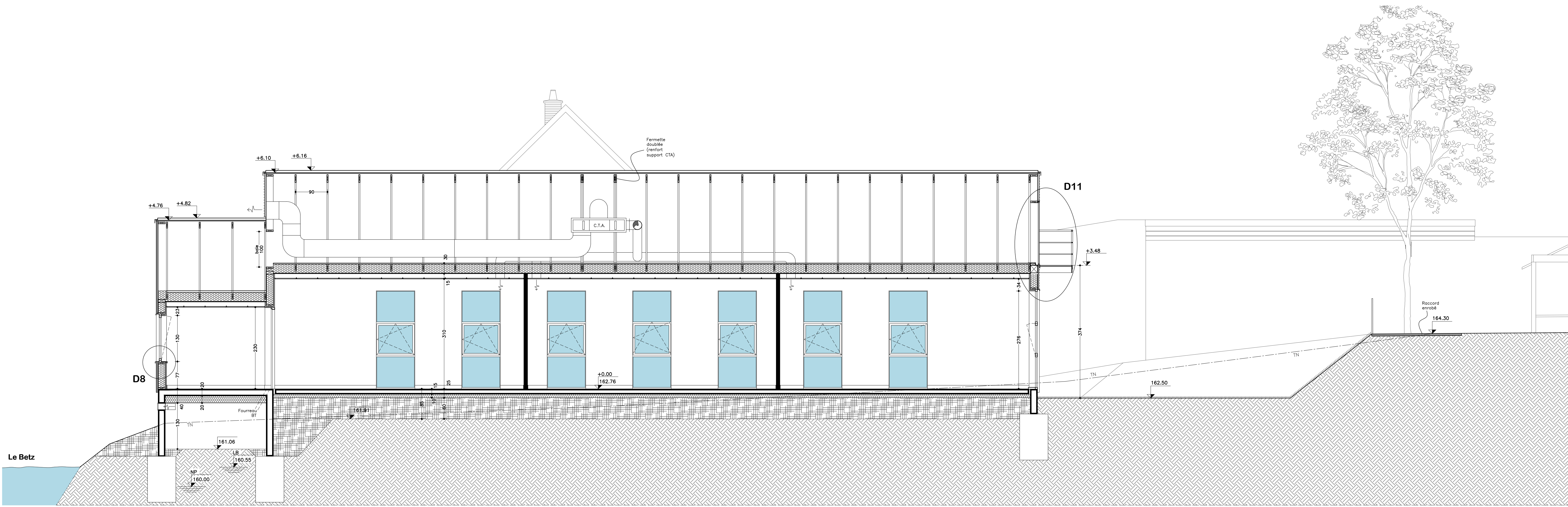
Coupe A
